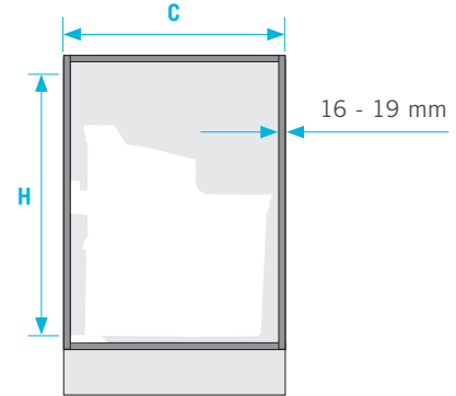
Önden görünüm
