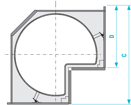
Üstten görünüm
