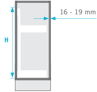
Önden görünüm
