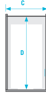
Üstten görünüm
