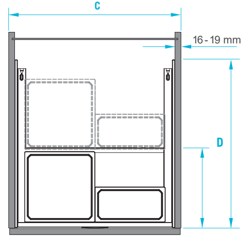
Üstten görünüm
