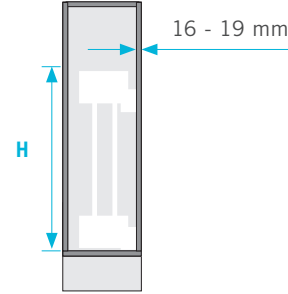
Önden görünüm
