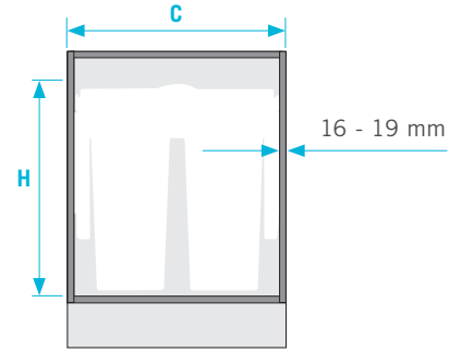
Önden görünüm
