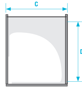
Üstten görünüm
